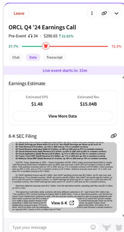
Data Tab
