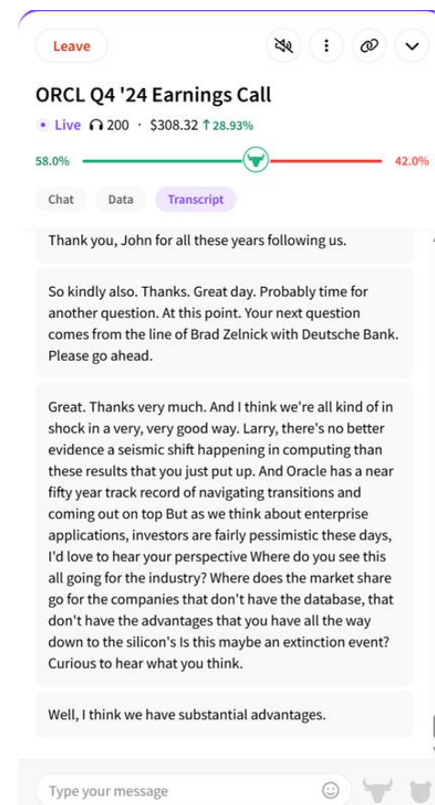
Transcript Tab
