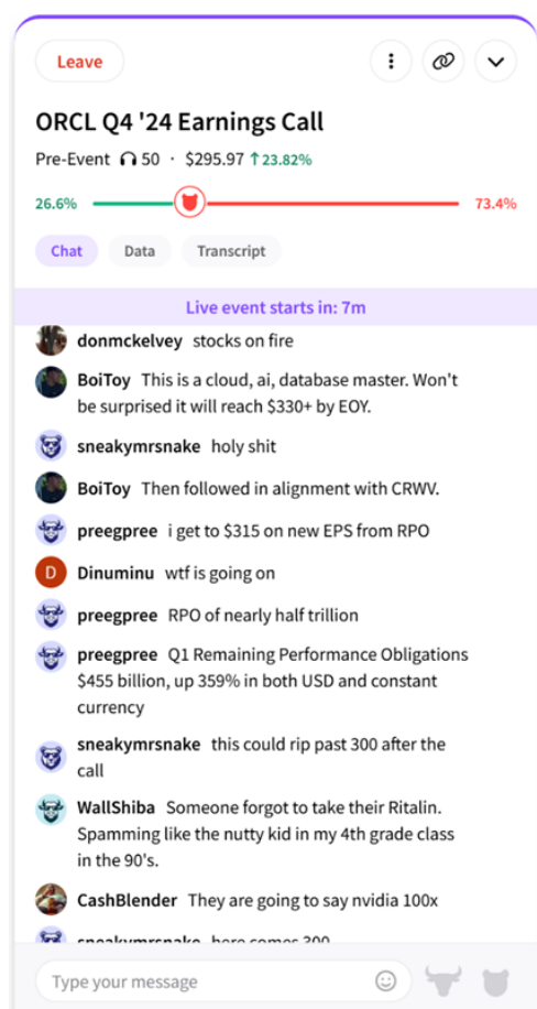
Chat Tab
